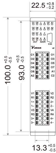
主视图
