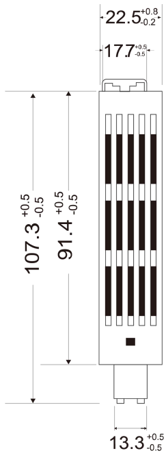
俯视图
